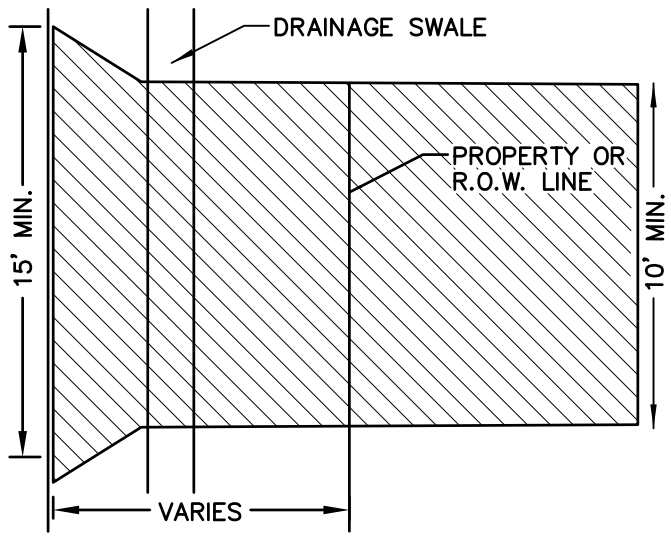
PLANVIEW N.T.S.
